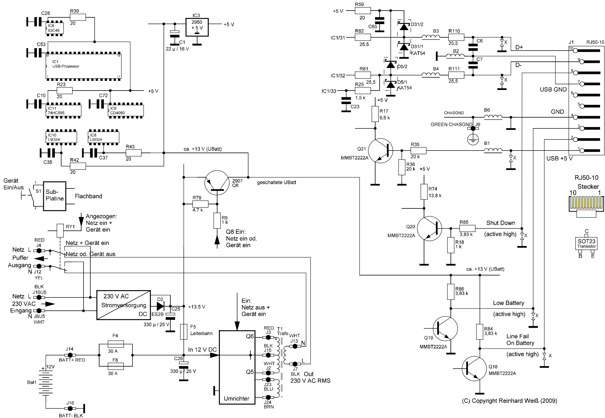
Basisplatine (Teilbereich) APC Back-UPS CS 350 (640-0287E_REV14)
